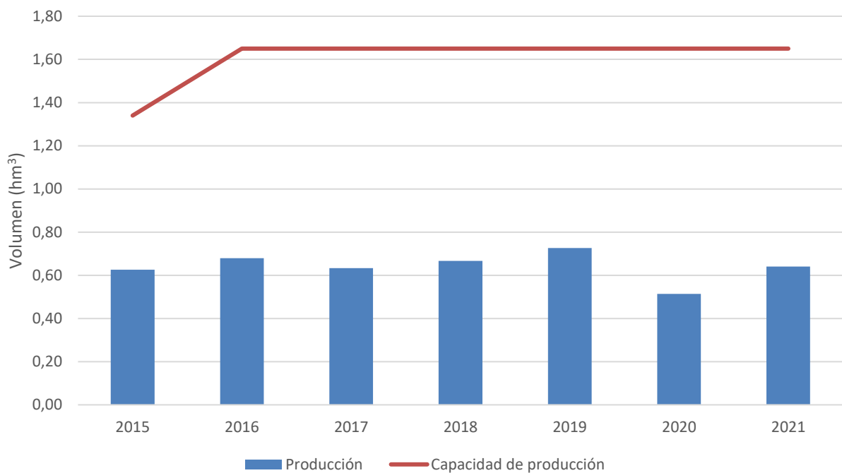
Figura 8. Producción y capacidad de producción de agua desalada en Formentera. Elaboración propia (Fuente: ABAQUA).
