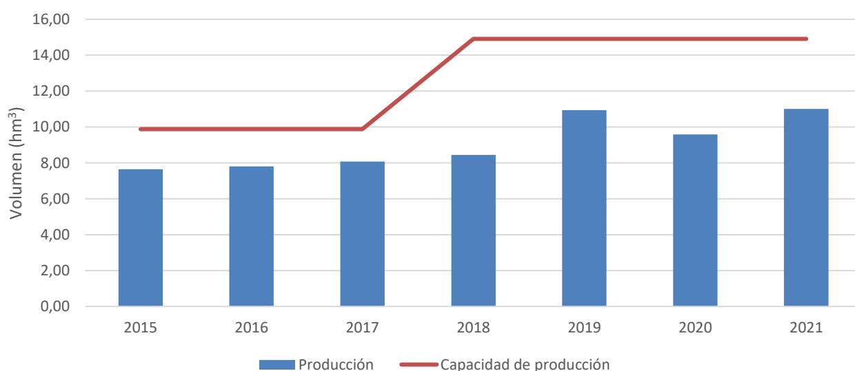
Figura 7. Producción y capacidad de producción de agua desalada en la isla de Ibiza. Elaboración propia (Fuente: ABAQUA).
