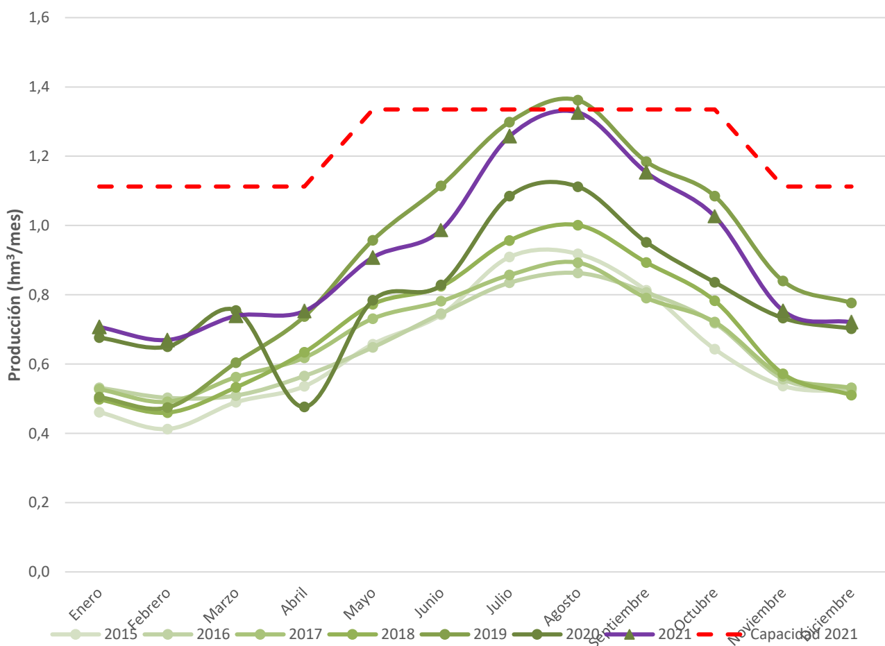
Figura 9. Producción de agua desalada en la isla de Ibiza por meses. Elaboración propia (Fuente: ABAQUA).
